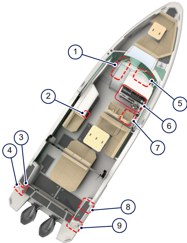
Kuva 4.8 - Käyttäjän hallintalaitteiden sijainnit
