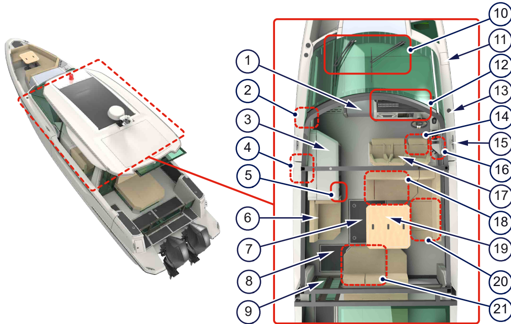
Kuva 4.4 - Ohjaamo
