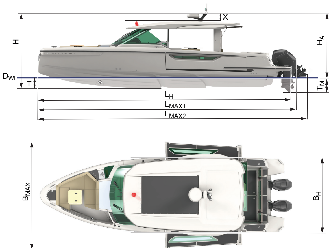
Kuva 8.1 - Saxdor 400 GTO:n mitat
