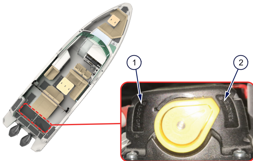
Kuva 5.3 - Akkupaketin turvarelekytkin
