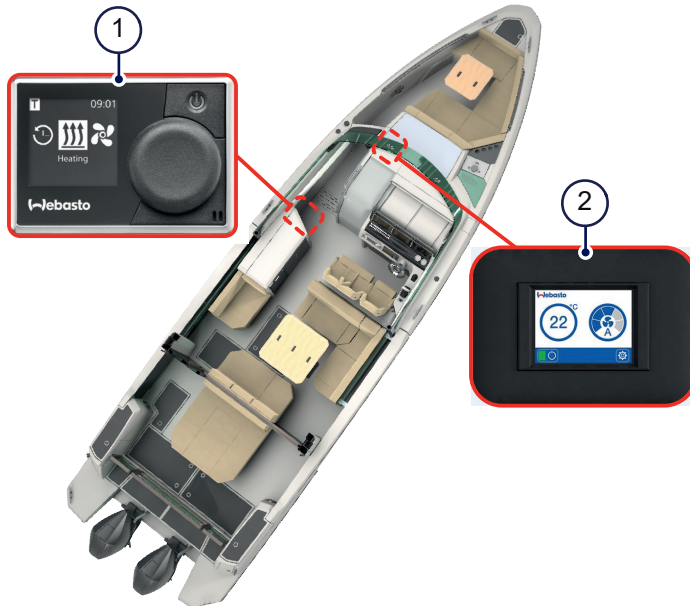
Kuva 4.18 - Lämpötilan ohjauspaneeli
