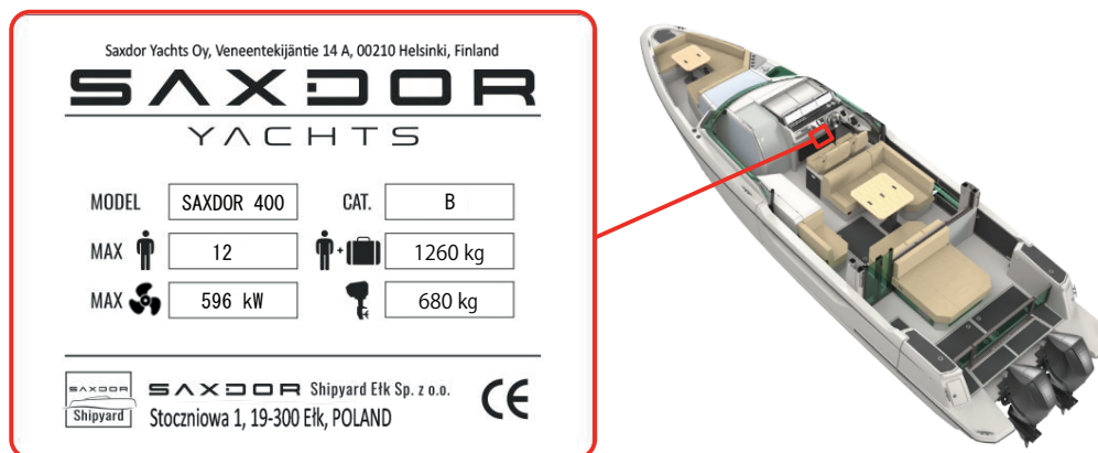
Kuva 4.19 - Valmistajan kilpi
