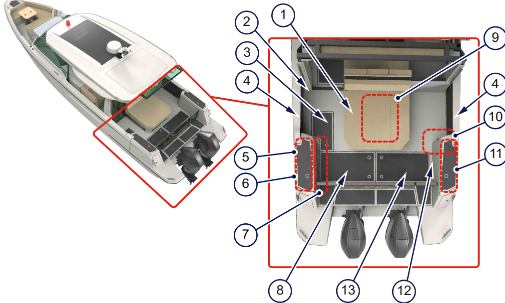
Kuva 4.6 - Peräkansi
