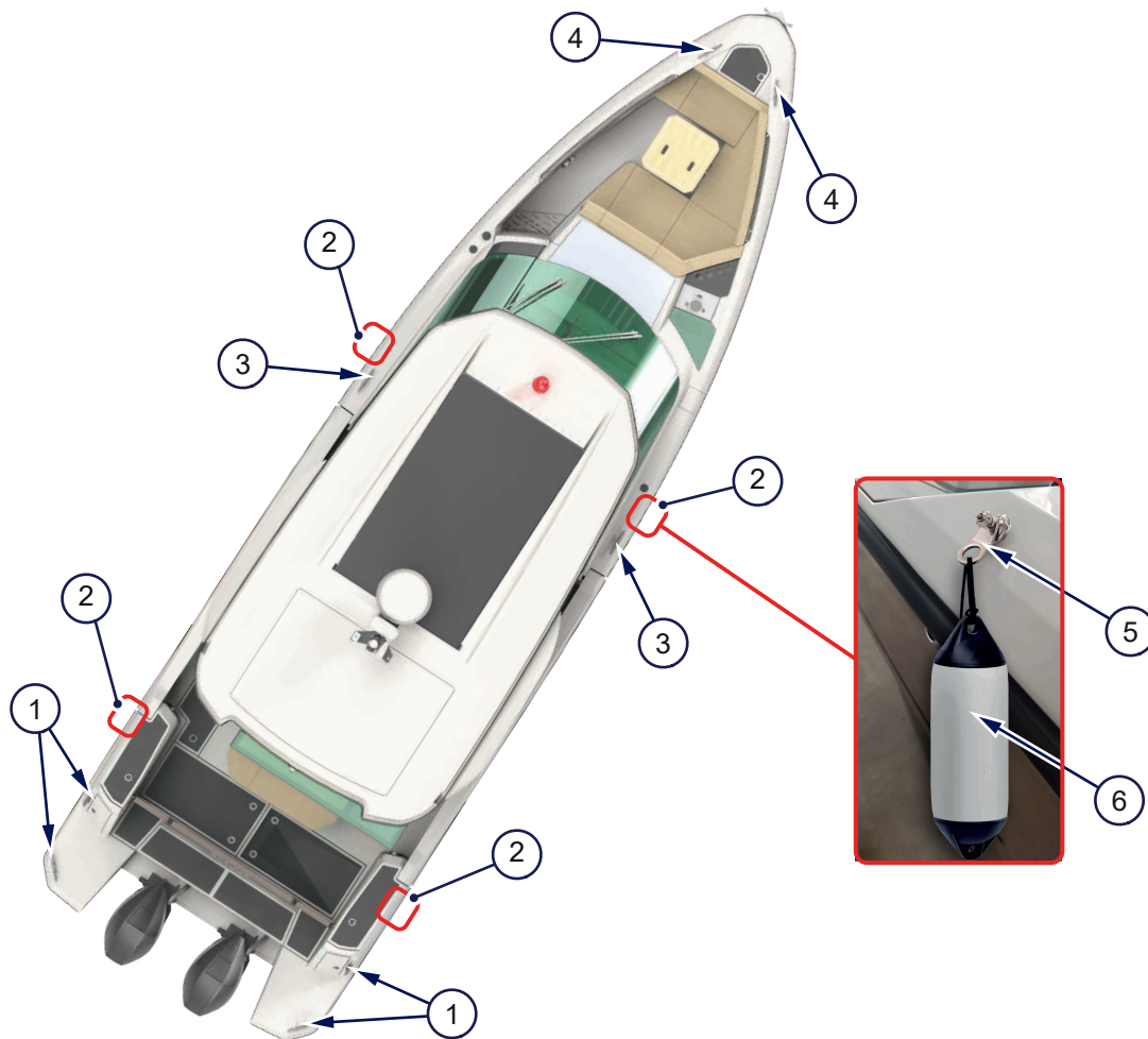
Kuva 4.23 - Kiinnityskohdat
