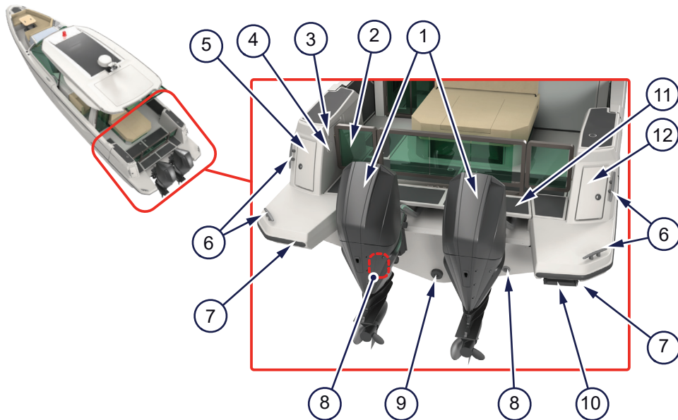
Kuva 4.7 - Uimatasanne
