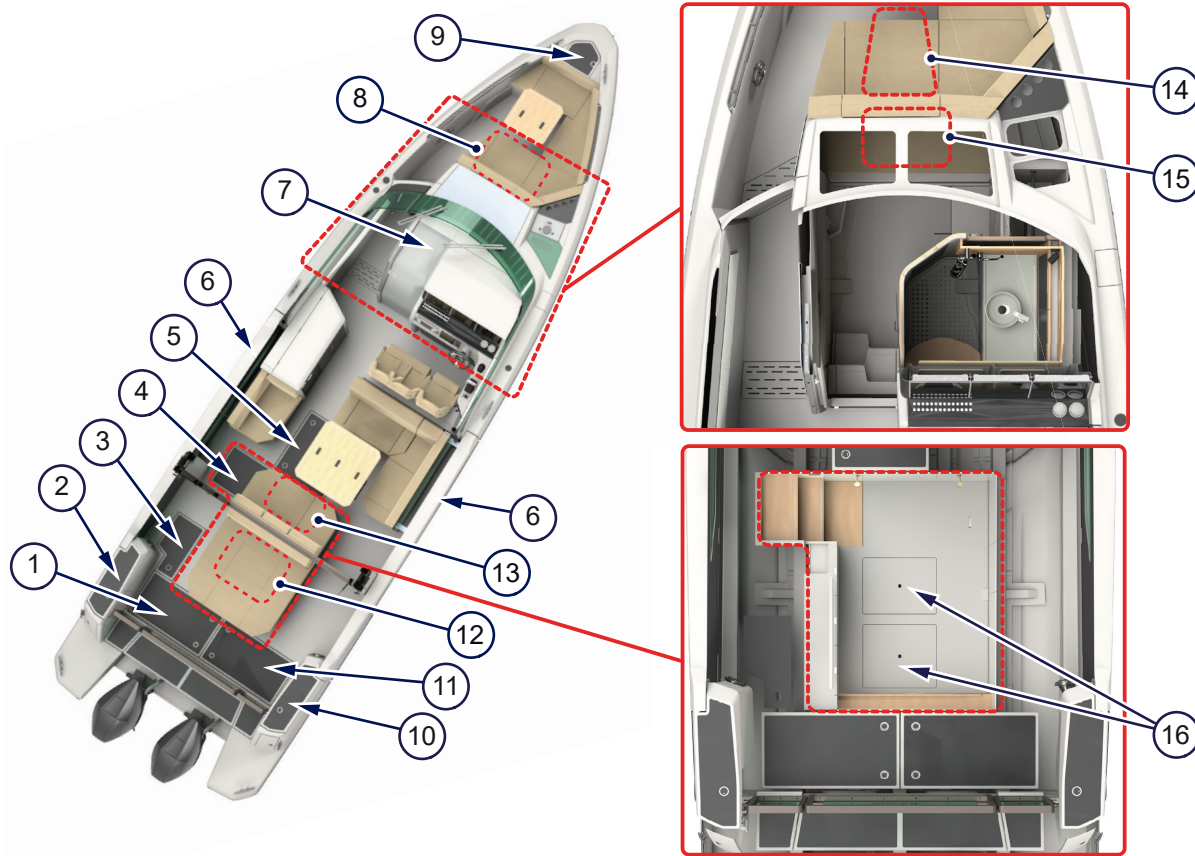
Kuva 4.26 - Luukut
