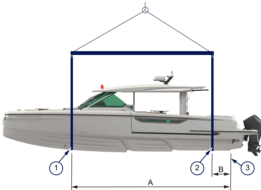
Kuva 4.24 - Nostopisteet
